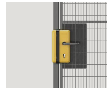
CERRADURA DE BOMBÍN EURO Con espacio para un interruptor de seguridad sin contacto integrado.
