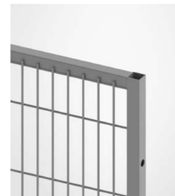
PANEL DE MALLA ST20 El panel de malla ST20 tiene un diseño clásico con una luz de malla de 20x100 mm fijado a un marco de 19x19 mm. Disponible en tres alturas estándar, 1.250, 2.050 y 2.350 mm en hasta 8 anchos.
